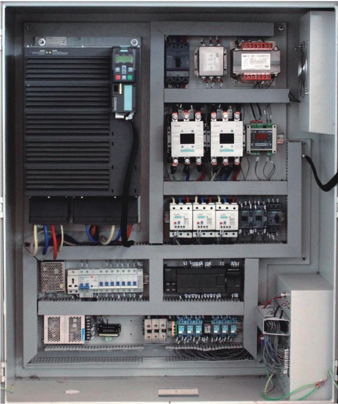
变频梯控制系统
